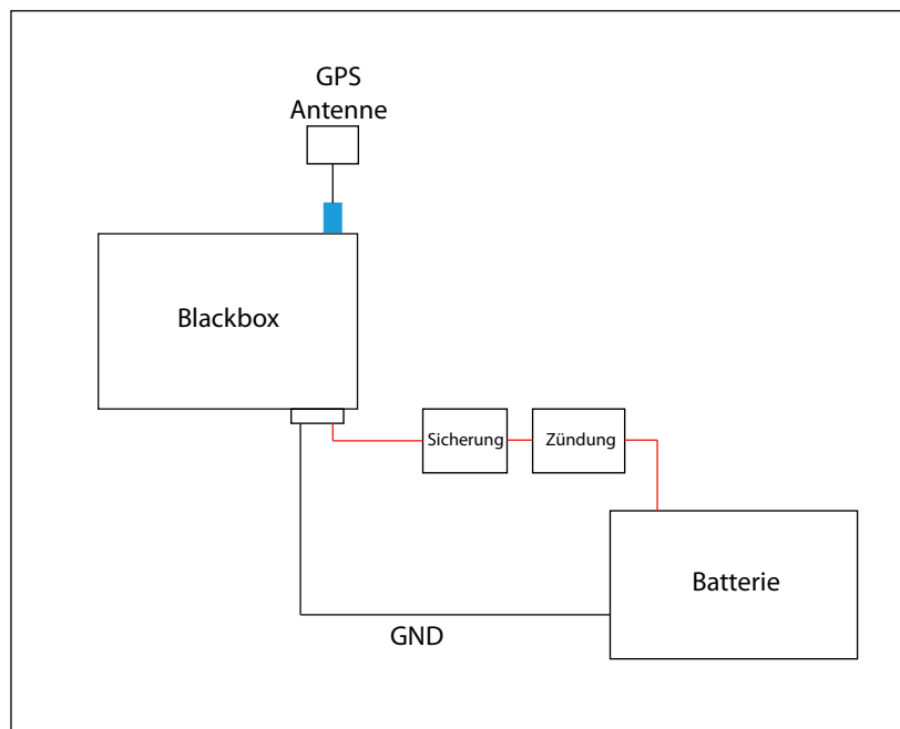
Installationsschema
